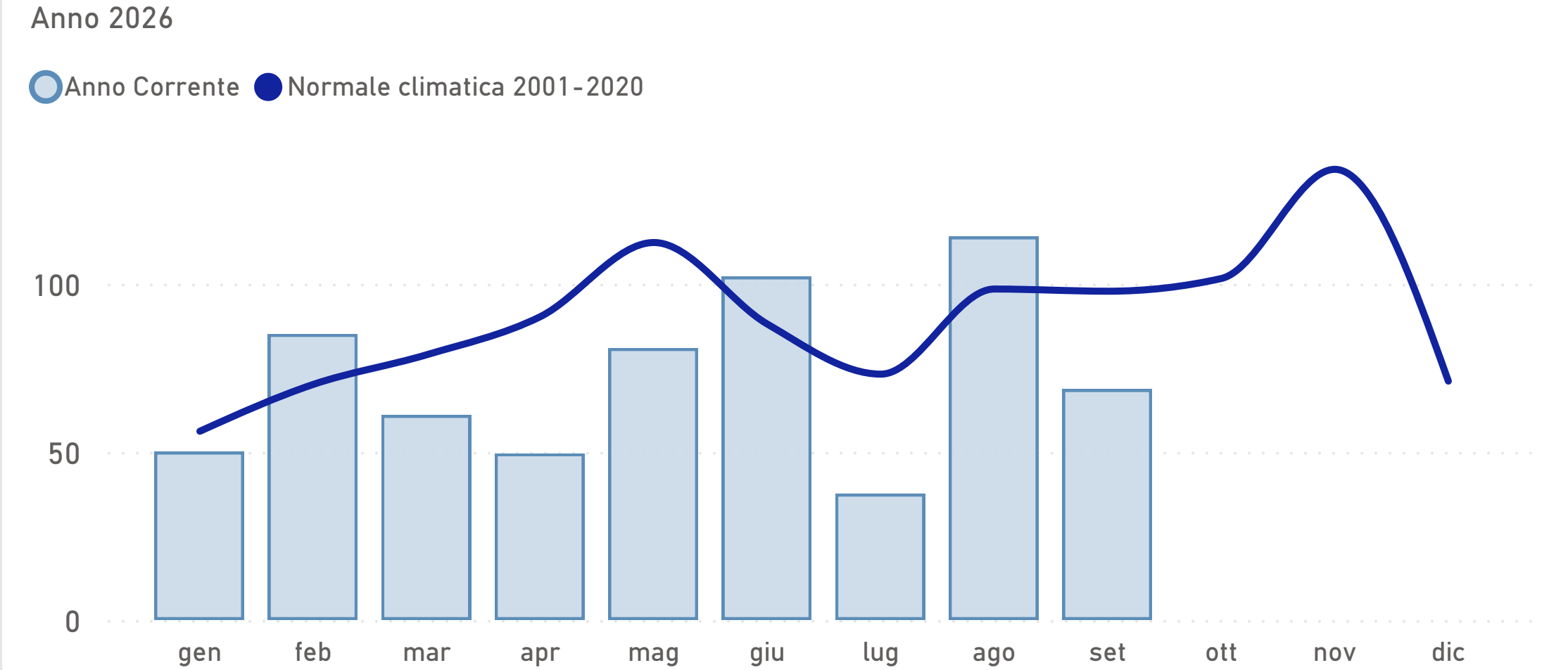
Precipitazioni Totali Mensili (mm) - Confronto con Normale Climatica 2001-2020
