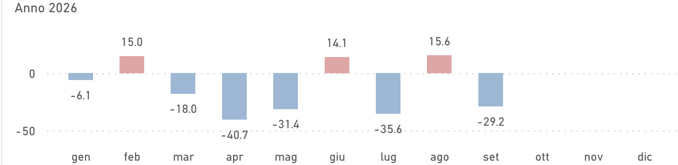
Anomalia vs Normale Climatica (mm) per Mese
