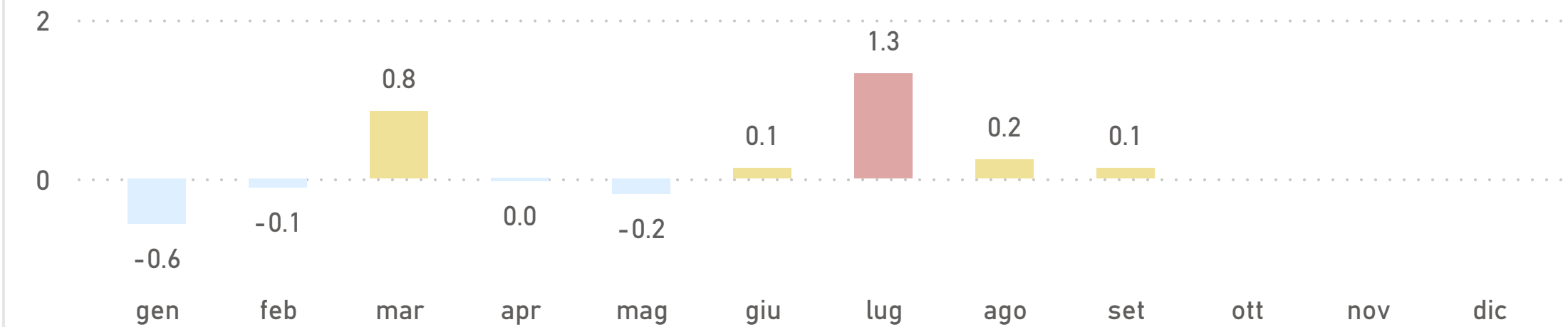
Anomalia vs Normale Climatica (km/h) per Mese
